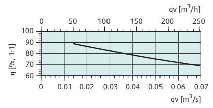
Температурная эффективность
