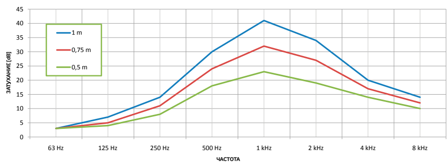
Затухание шумоглушителей
