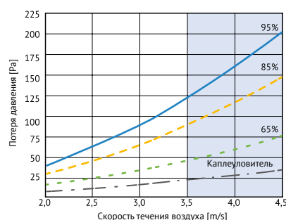
Потеря давления
