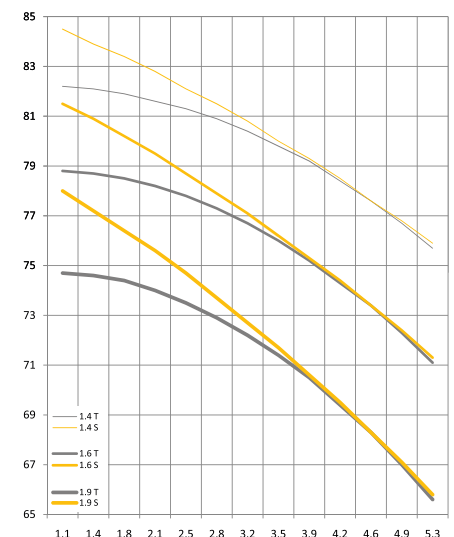
Тепловое к.п.д. (%) в зависимости от скорости течения воздуха (m/s) и типа ротора
