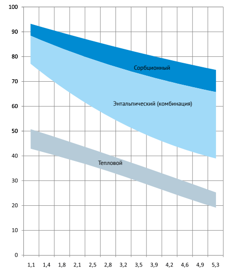
Потеря давления (Pa) в зависимости от скорости течения воздуха (m/s) и типа ротора
