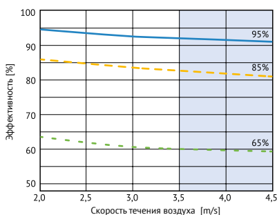
Эффективность увлажнения
