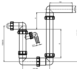
Сифон, предварительно заполняемый водой
